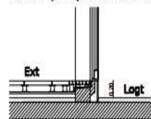
Schéma principe accès extérieur
